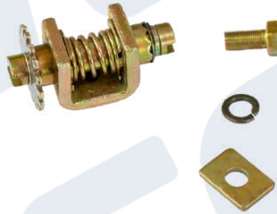
FREN AYAR MEKANİZMASI EM. ORJİNAL NO : 8528686 MODEL : 50 NC
